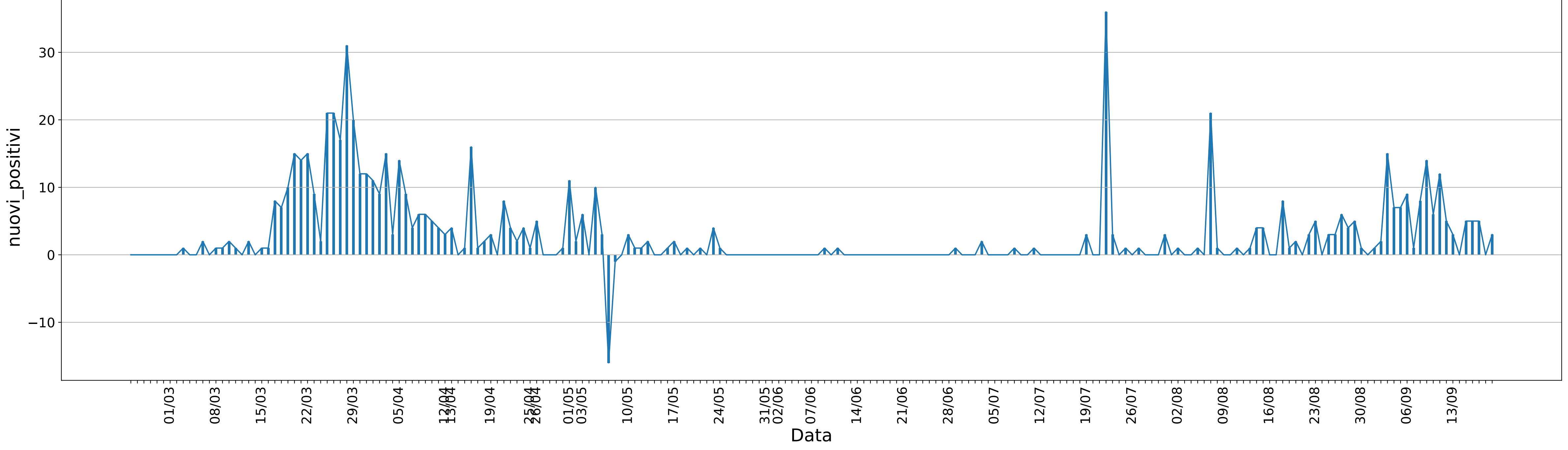
nuovi_positivi per la regione Basilicata
