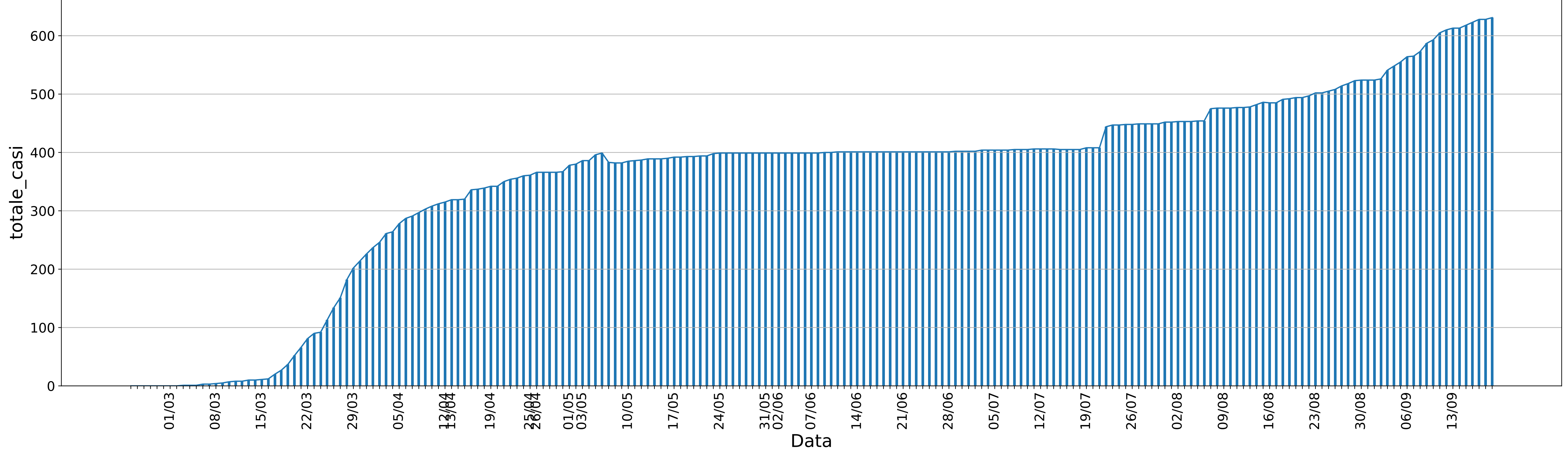
totale_casi per la regione Basilicata
