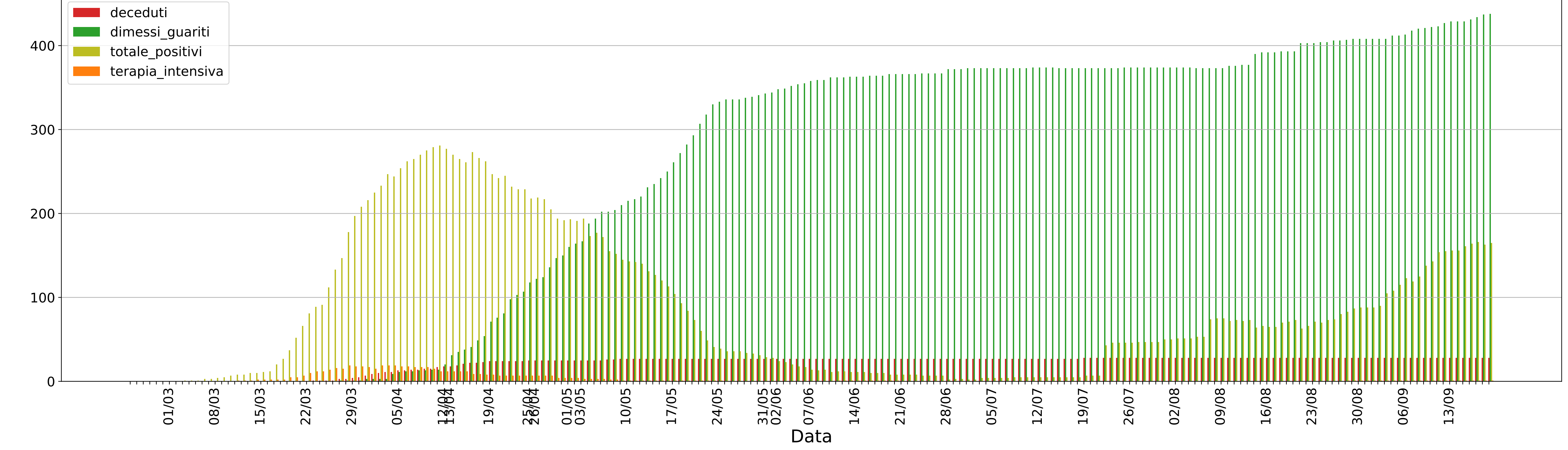
Confronto andamenti deceduti/dimessi_guariti/totale_positivi/terapia_intensiva per la regione Basilicata
