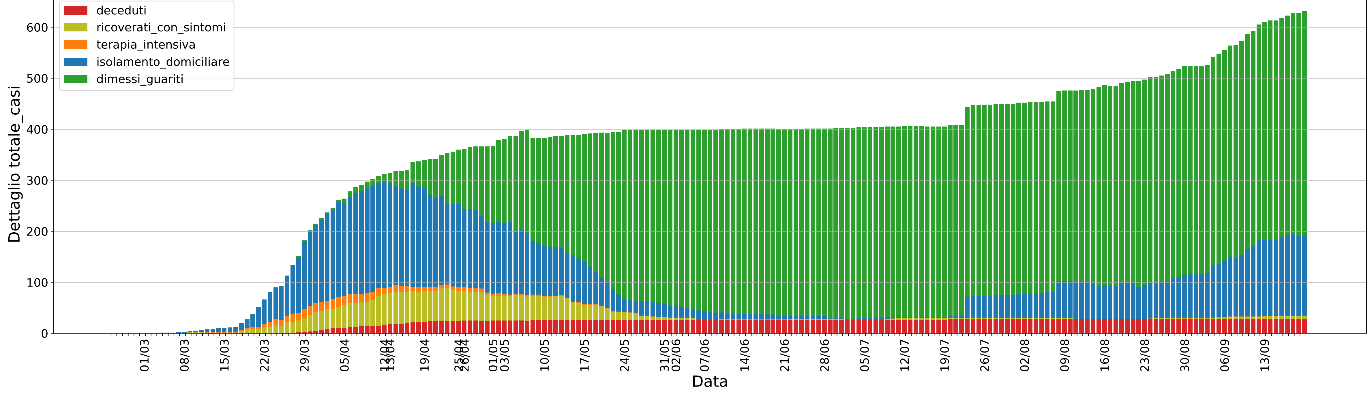
Confronto andamenti deceduti/ricoverati_con_sintomi/terapia_intensiva/isolamento_domiciliare/dimessi_guariti per la regione Basilicata
