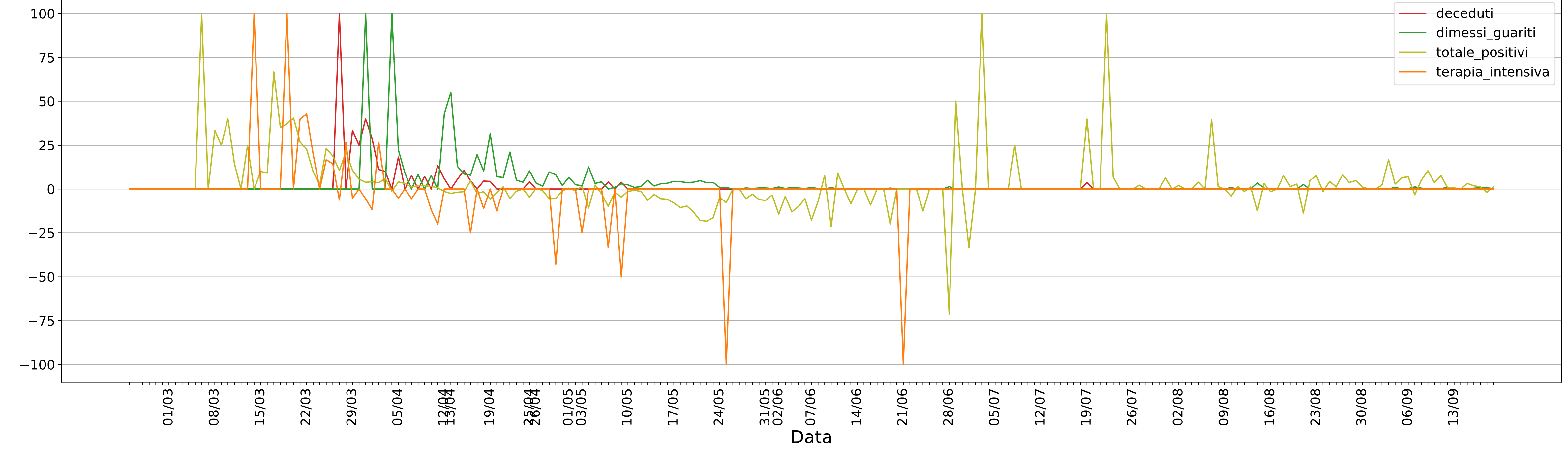
Variazione % rispetto alla giornata precedente di deceduti/dimessi_guariti/totale_positivi/terapia_intensiva
